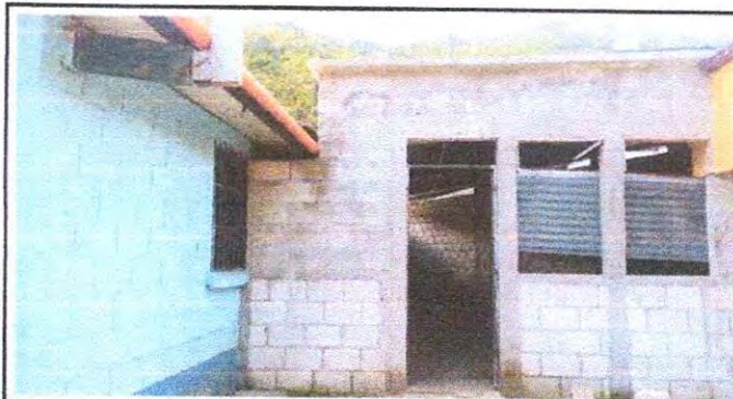
foto: 6 Colocacion de puertas y ventanas de la cocina.
